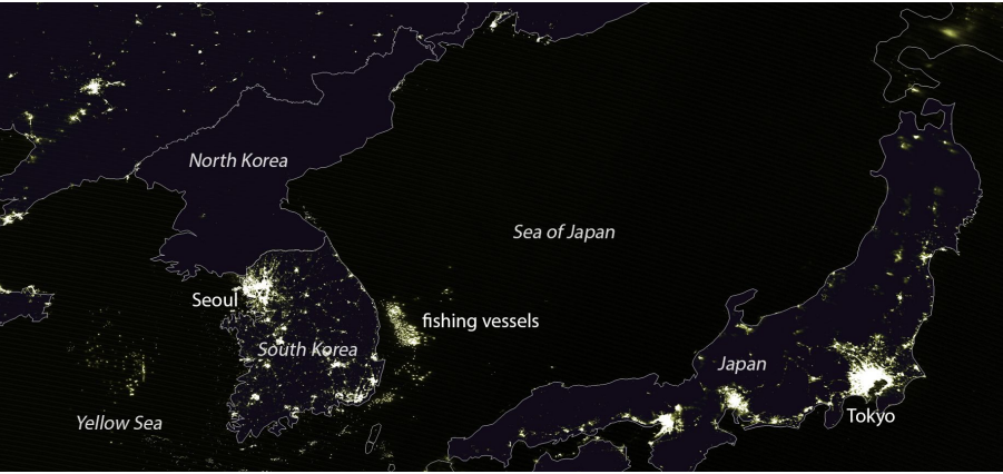
VIIRS
